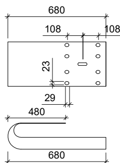
TERMINAL CON RETORNO BIONDA SIMPLE
