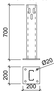
POSTE CPN120 CON PLACA 200x200x10
