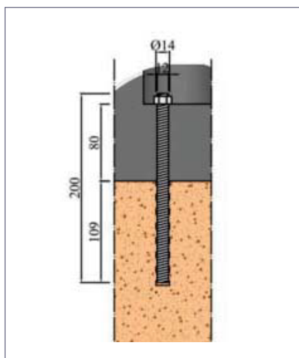
Fijaciones en el centro del separador.
