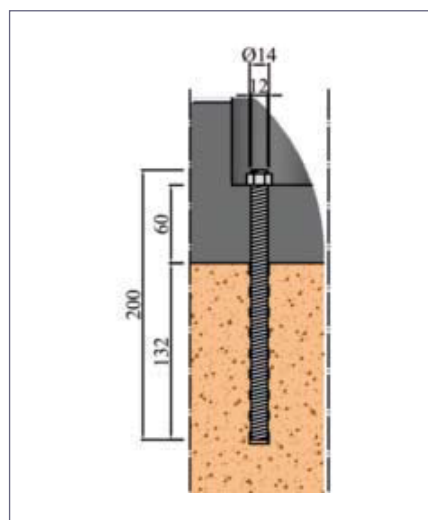
Fijaciones en los extremos del separador.
